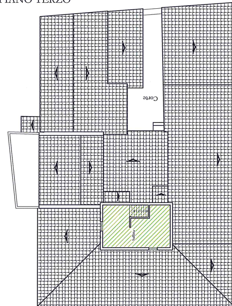
PIANO TERZO
